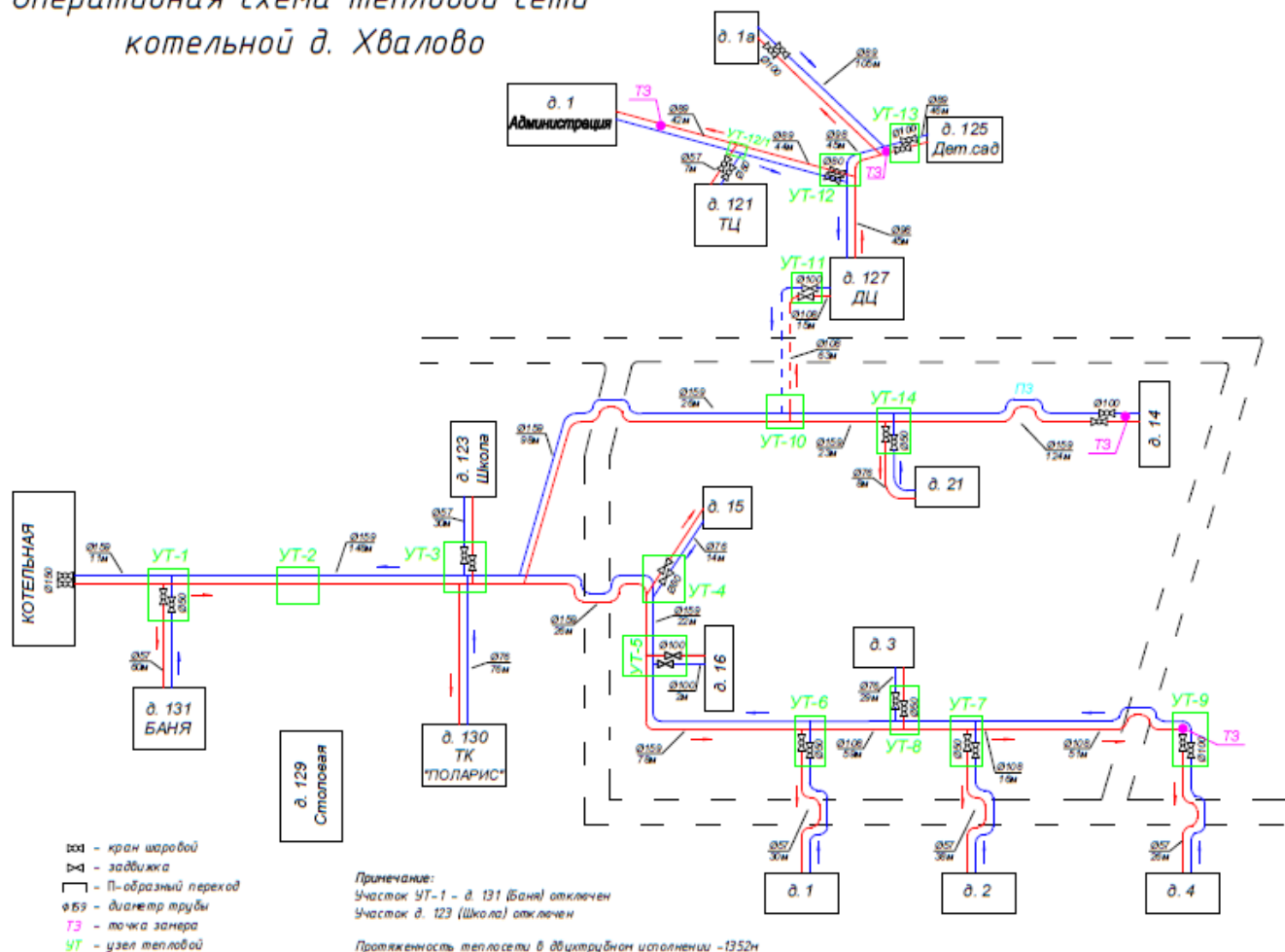
Рисунок 1 – Схема тепловых сетей в зоне действия Котельной д. Хвалово
